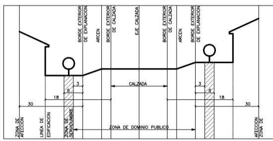
ZONA DE DOMINIO PÚBLICO, AFECTACIÓN Y SERVIDUMBRE EN SUELO RÚSTICO SECCIÓN TIPO CARRETERA AUTONÓMICA Y PROVINCIAL
